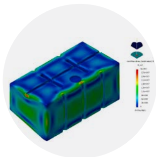
FEA SIMULACIJE DEFORMACIJ IN NAPETOSTI FEA DEFORMÁCIÓ- ÉS FESZÜLTÉGSZIMULÁCIÓ
